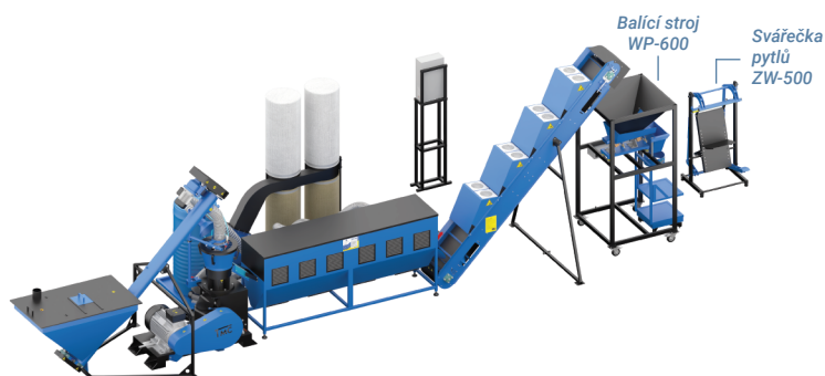
Linka na výrobu pelet LDG-4000 KOMBI + balící stroj WP-600 + svářečka pytlů ZW-500
