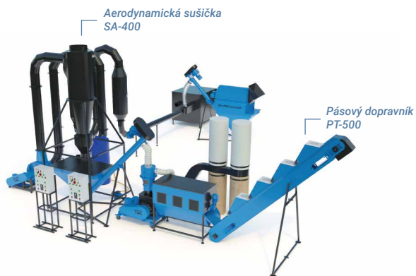
Linka na výrobu pelet LDG-2000 KOMBI + aerodynamická sušička SA-400 + pásový dopravník PT-500
