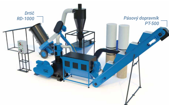
Linka na výrobu pelet LDG-3000 KOMBI + pásový dopravník PT-500 + drtič RD-1000 s cyklónem
