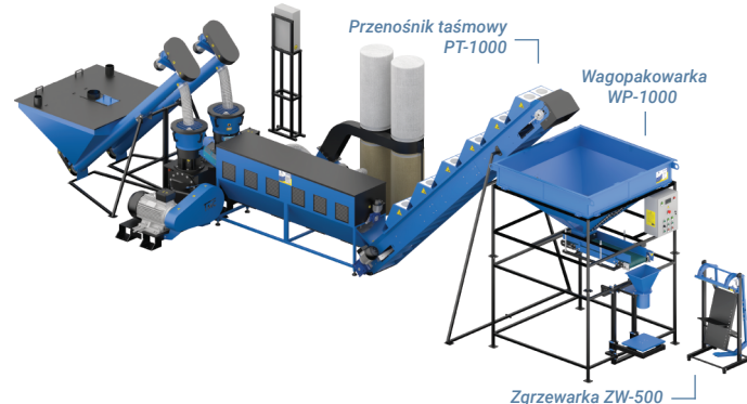
Linia do produkcji pelletu LDG-3000 DUO + Przenośnik taśmowy PT-1000 + Wagopakowarka WP-1000 + Zgrzewarka ZW-500
