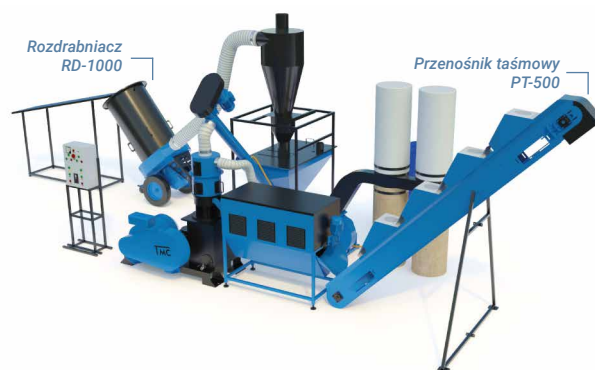
Linia do produkcji pelletu LDG-3000 KOMBI + Przenośnik taśmowy PT-500 + Rozdrabniacz RD-1000 z cyklonem
