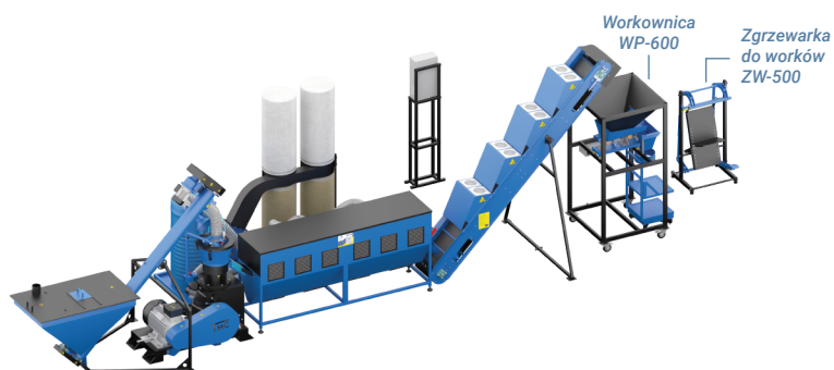
Linia do produkcji pelletu LDG-4000 KOMBI + Workownica WP-600 + Zgrzewarka do worków ZW-500
